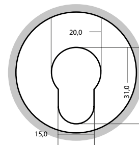
zámok A
