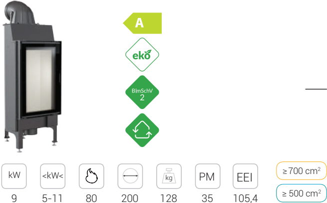
NADIA 12 606x1132x1034x449
