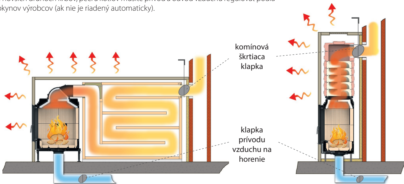
Ručná regulácia prívodu vzduchu a odvodu spalín z ohniska v modernej akumuláčnej kachľovej peci (vľavo) a v akumuláčnom krbe (vpravo).
